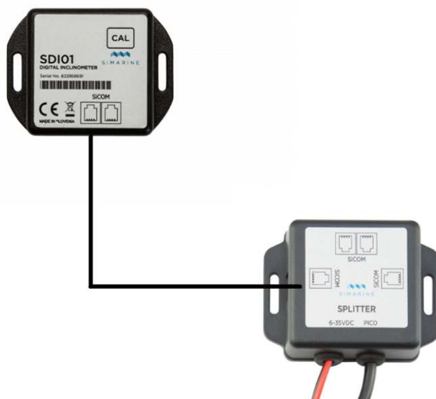
STANDARDVERKABELUNG - DIREKT ZUM SPLITTER
