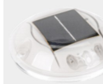
型号(model):LZL-DD-07 材料(material):铝(aluminium); 太阳能电池(solar battery) 尺寸(size):110×95×23mm
